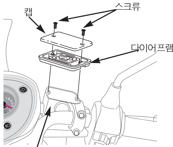
마스터실린더 보디
