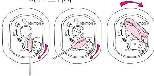
메인 스위치
