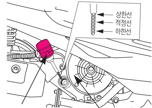
오일레벨게이지
