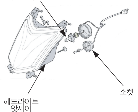
헤드라이트 벌브
