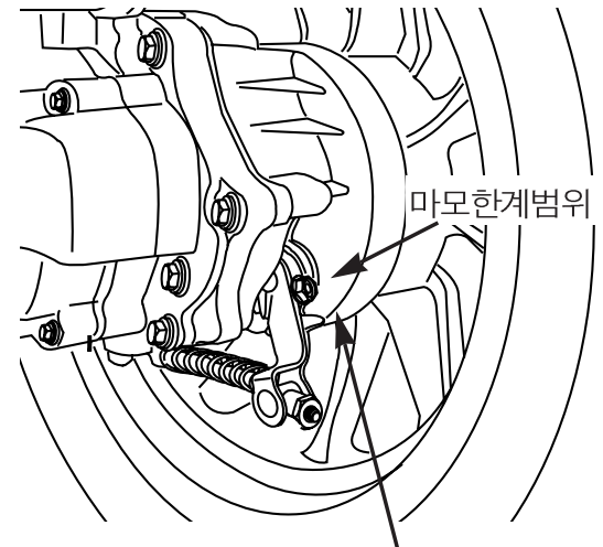
브레이크암 인디케이터
