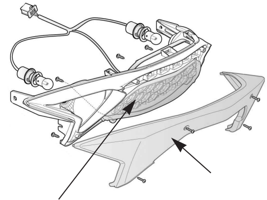
리어 콤비라이트 (LED) 앗세이
