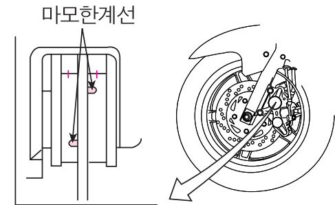
[전륜]
