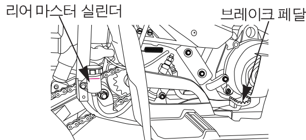
(전륜/후륜 브레이크)
