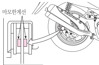
후륜
