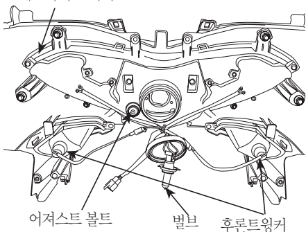
헤드라이트 커버
