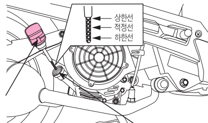
오일레벨게이지
