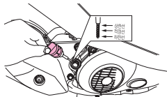
(엔진 오일량)
