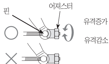
리어 브레이크 슈의 점검
